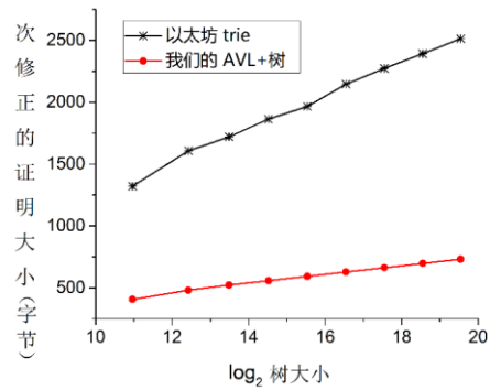
图 1: 尔格的AVL+ 树和 Merkle patriciatrie的证明大小比较
